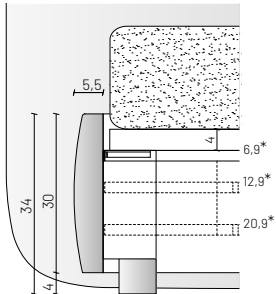
rete regolabile su tre altezze adjustable slats on three heights
