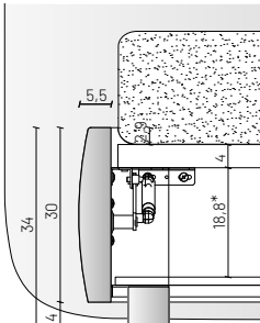
contenitore storage box
