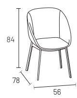
poltroncina imbottita A upholstered armchair A
