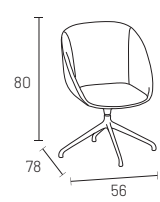
poltroncina imbottita B upholstered armchair B
