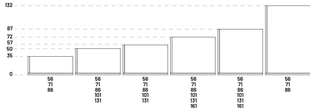
MODULARITÀ MODULI SLIM CASE MODULARITY OF SLIM CASE UNITS
