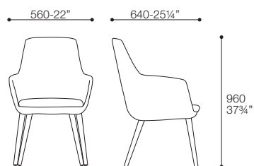
poltroncina Lyra con braccioli /Lyra armchair with armrests
