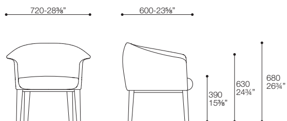
poltroncina Milo /Milo armchair
